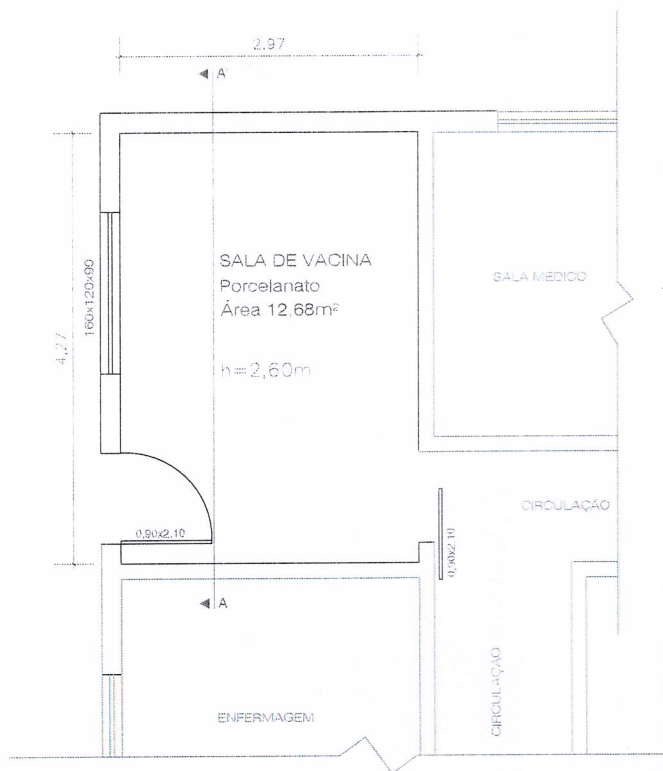
PLANTA BAIXA ESCALA 1/75
