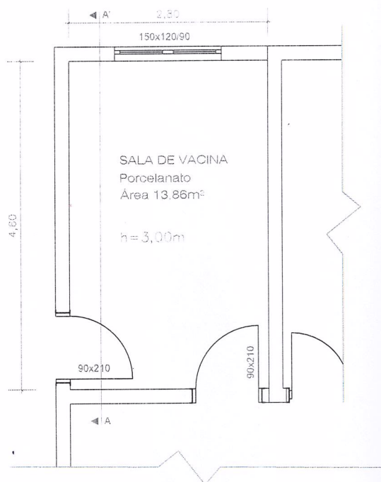
PLANTA BAIXA ESCALA 1/75
