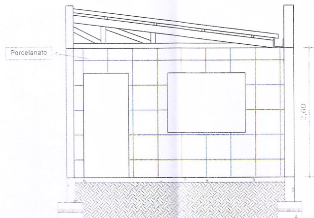
PLANTA DE CORTE ESCALA 1/75
