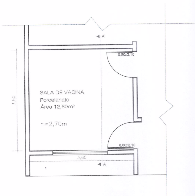
PLANTA BAIXA ESCALA 1/75
