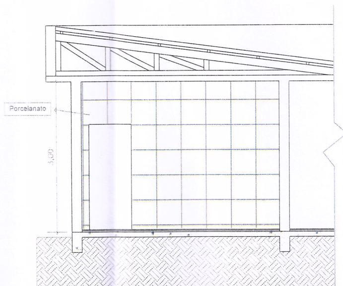
PLANTA DE CORTE ESCALA 1/75
