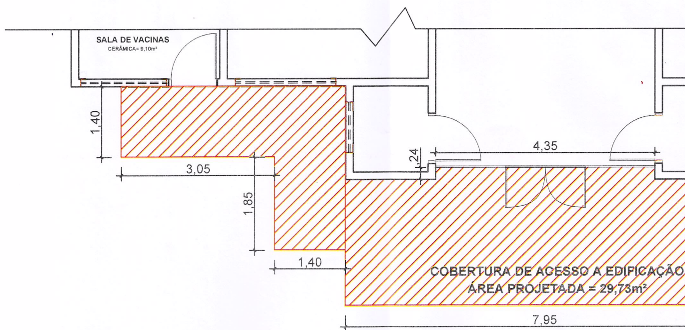
PLANTA DE IMPLANTAÇÃO Área: 29,73m² ESC.: 1:75
