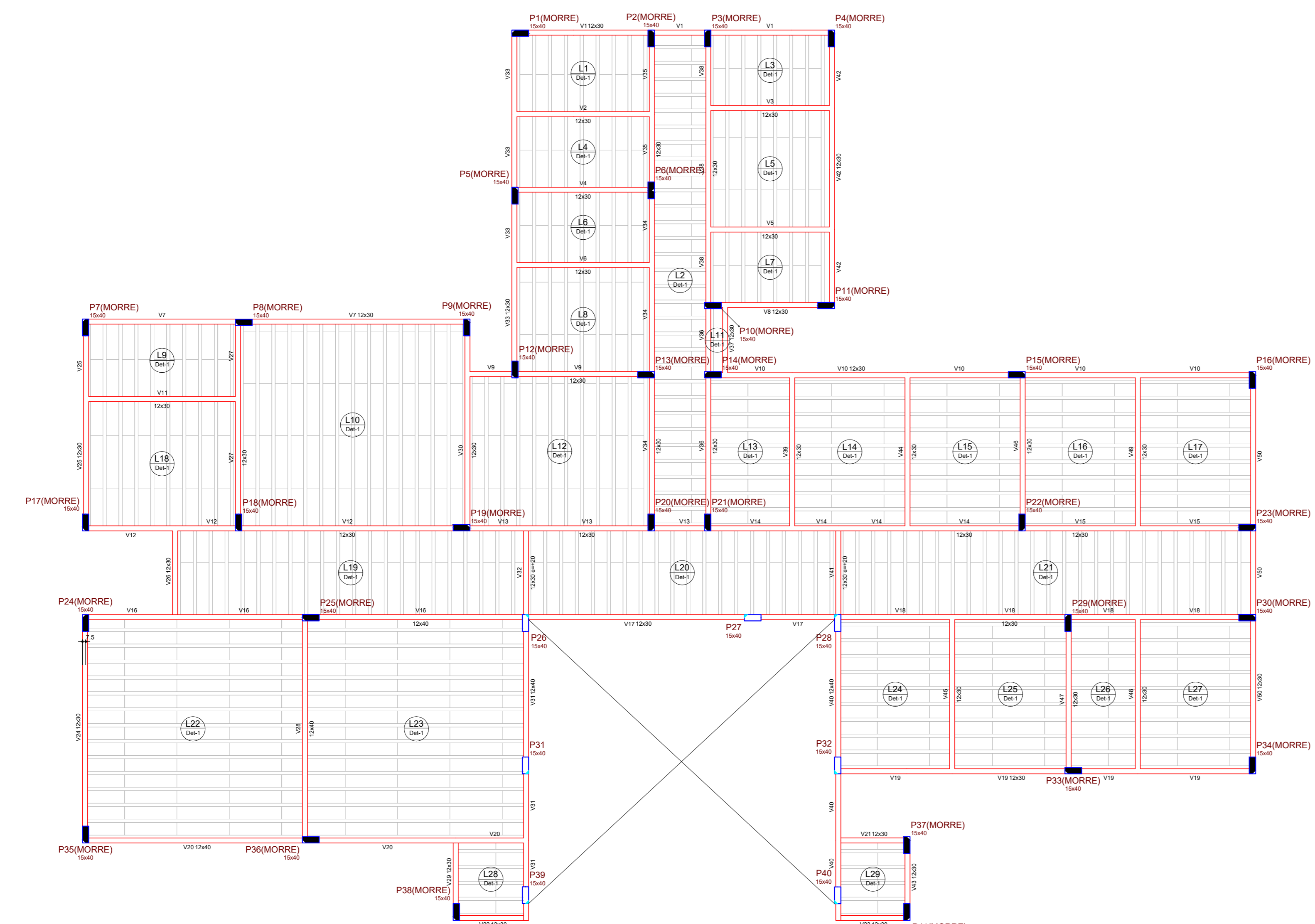
Forma do pavimento Cobertura escala 1:75
