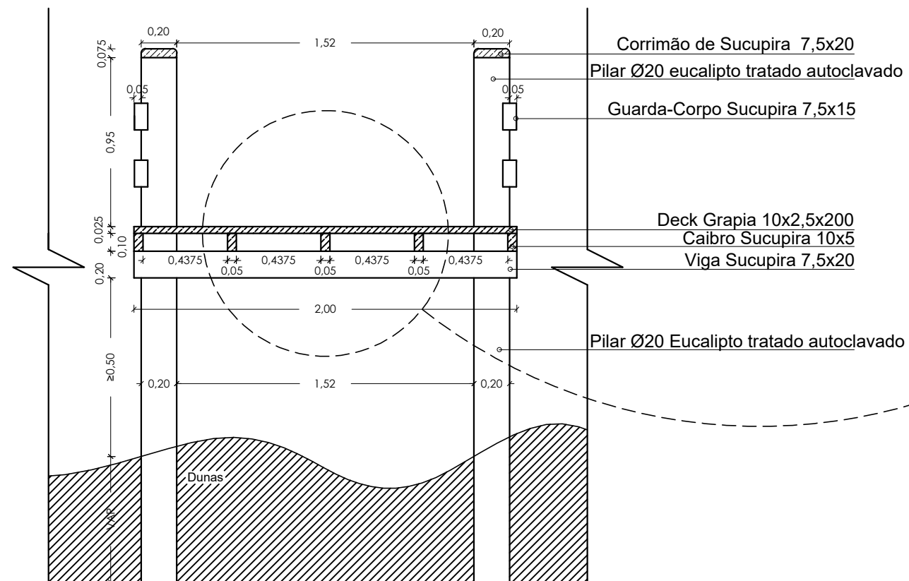
Corte Transversal esc 1:30
