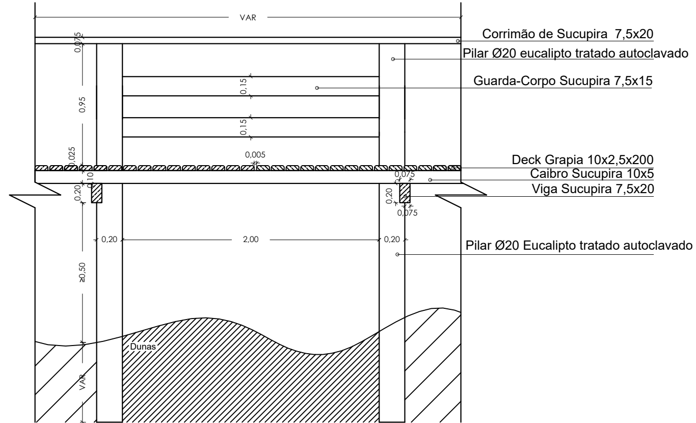
Corte Longitudinal esc 1:30
