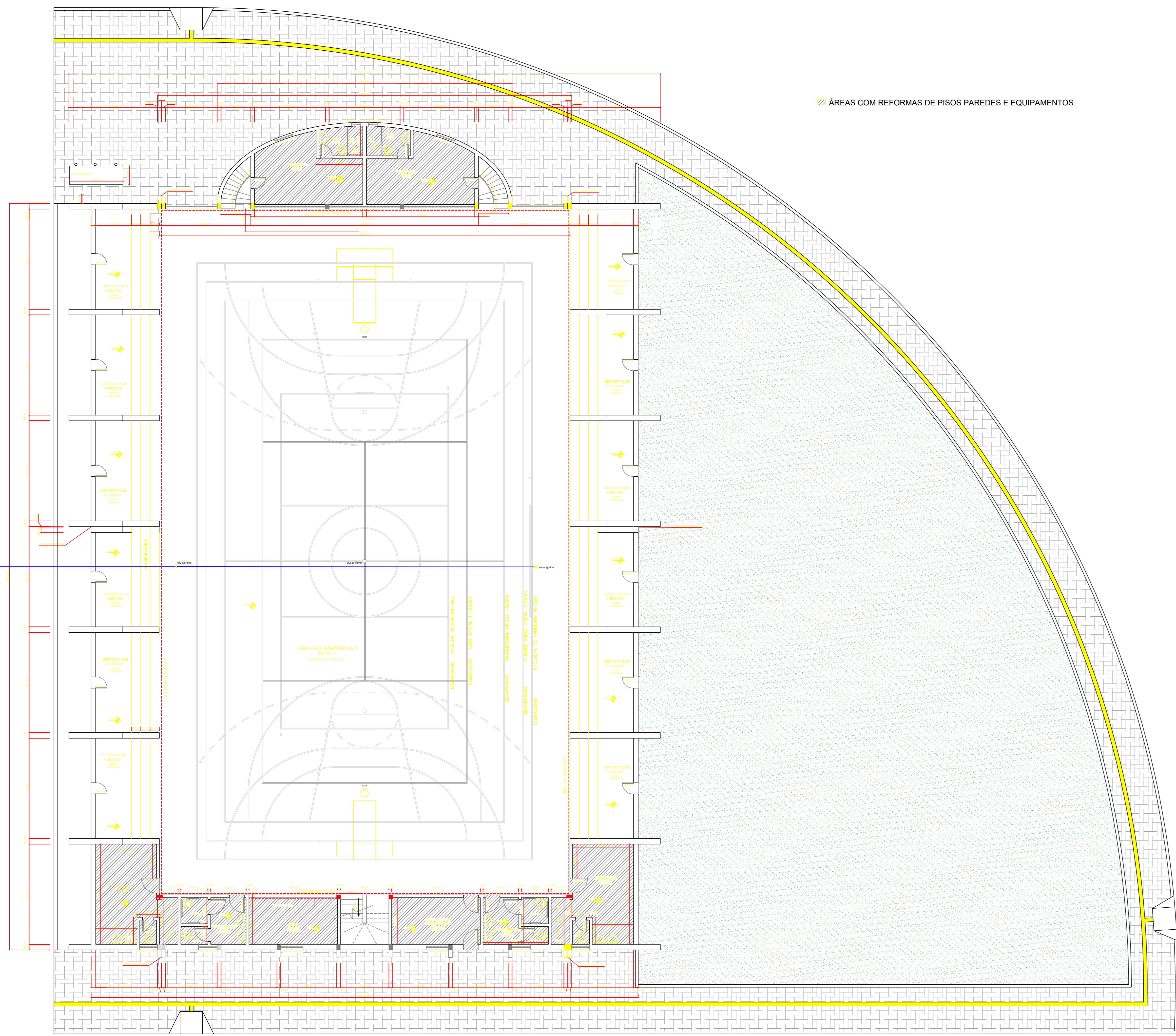
PLANTA BAIXA 1º PAVIMENTO ESC. 1:100
