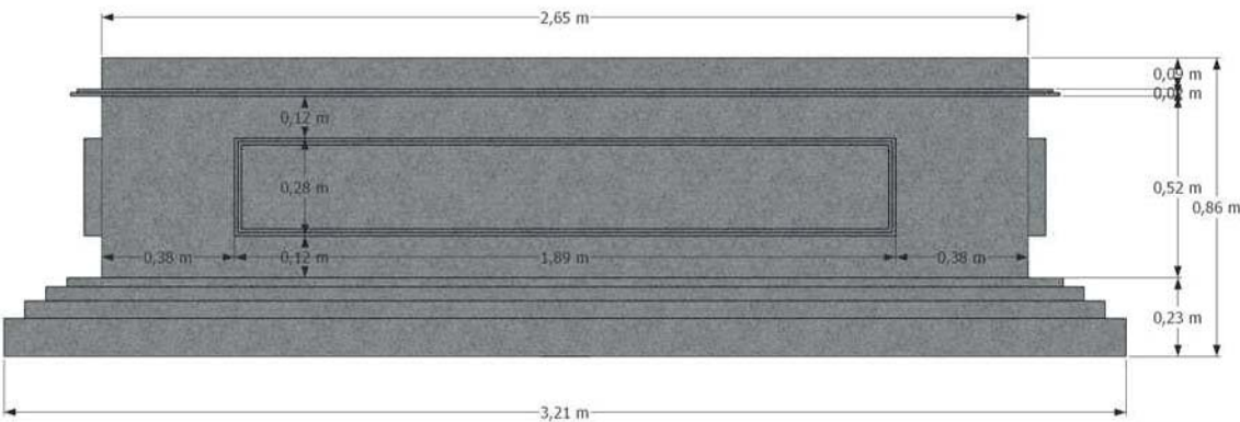
VISTA LATERAL SEM ESCALA
