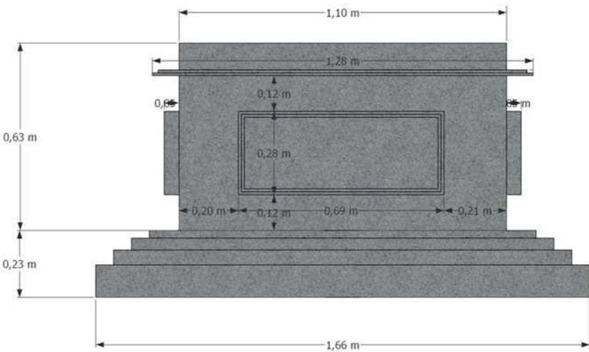
VISTA FRONTAL SEM ESCALA
